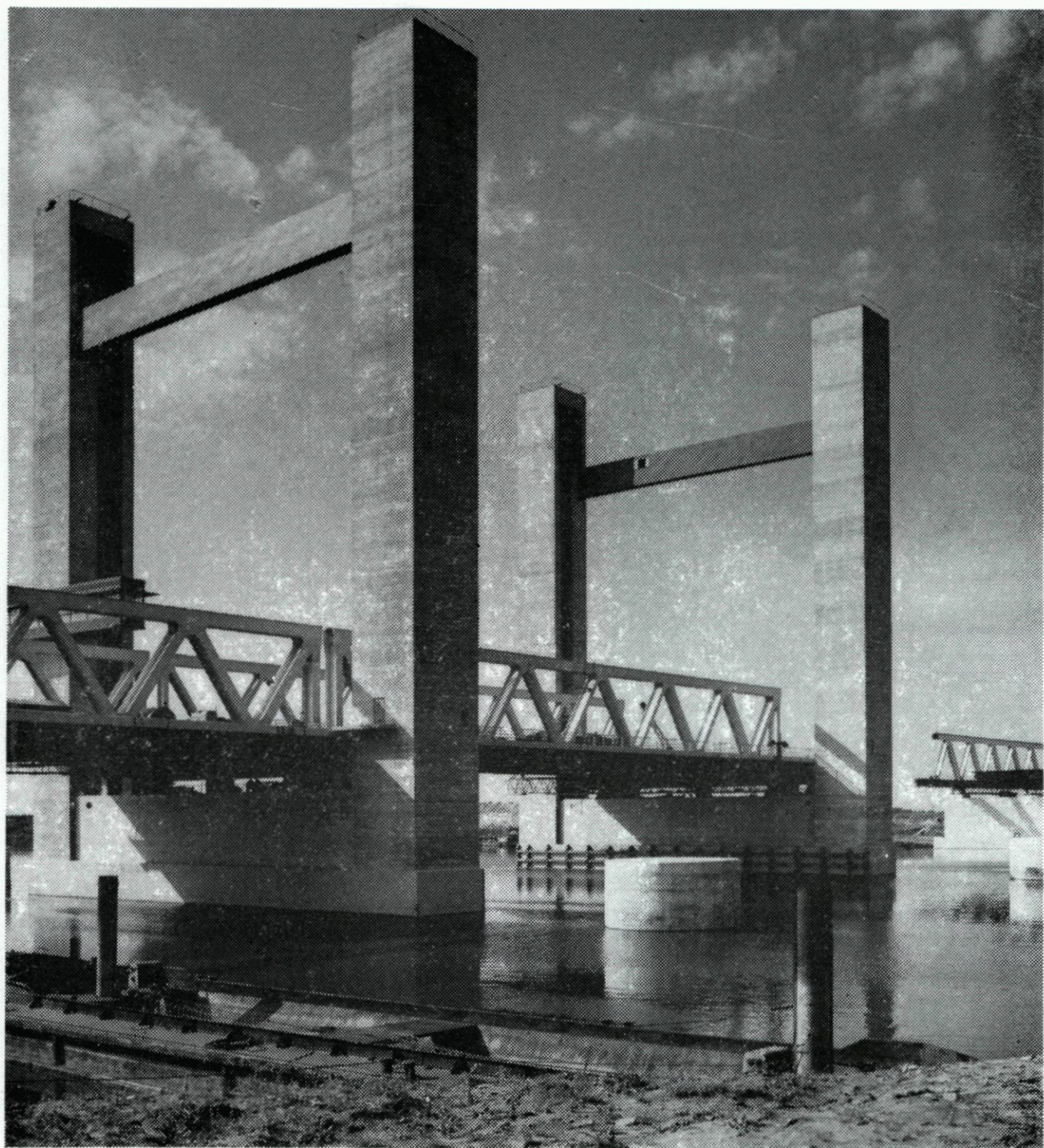
30. Calandbrug, gezien uit het noordoosten (JR).
