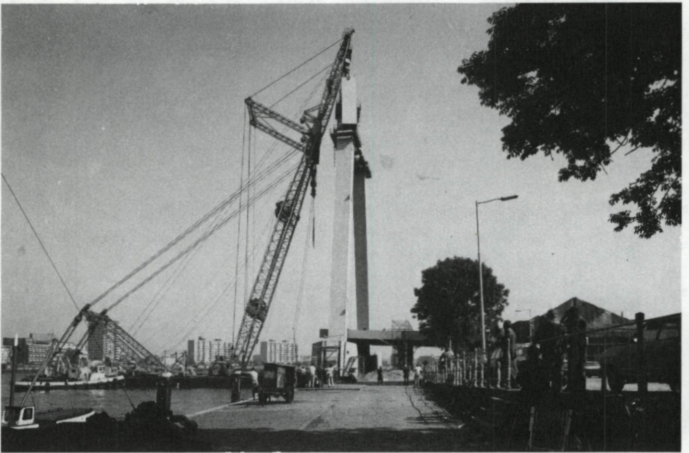
26-27. Het sluitstuk van de eerste pyloon van de in aanbouw zijnde Willemsbrug wordt aangebracht op de beide poten van de pyloon op de Maaskade, 29 augustus.
