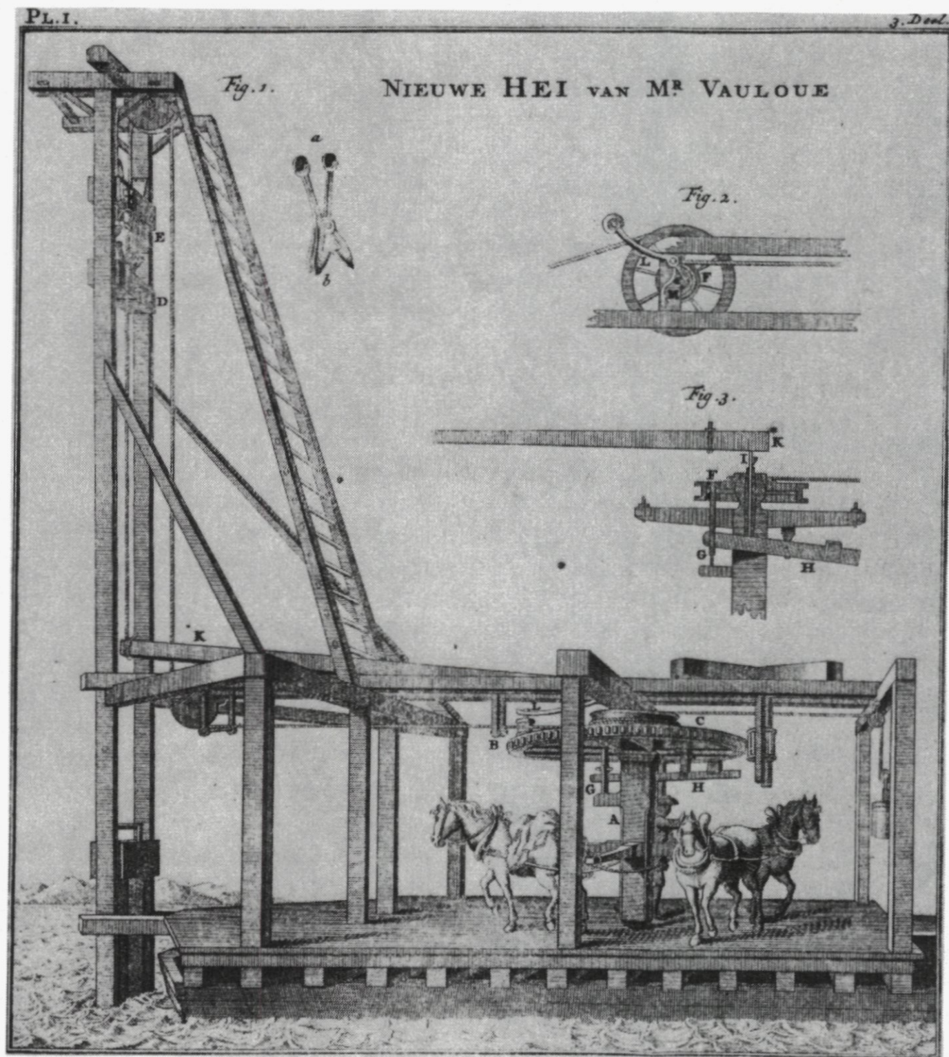
86. Tekening van de heimachine van Vauloué.
