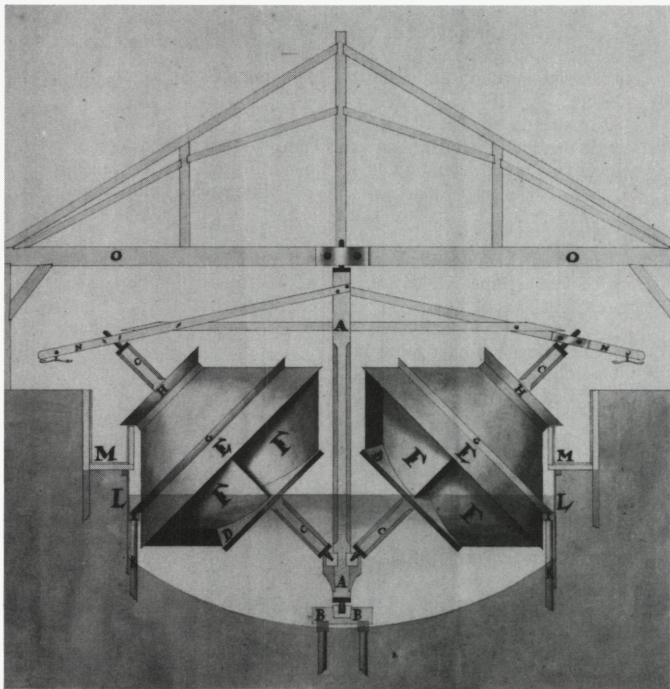
87. Tekening van de watermachine van Jacob van de Werken, 1782.
