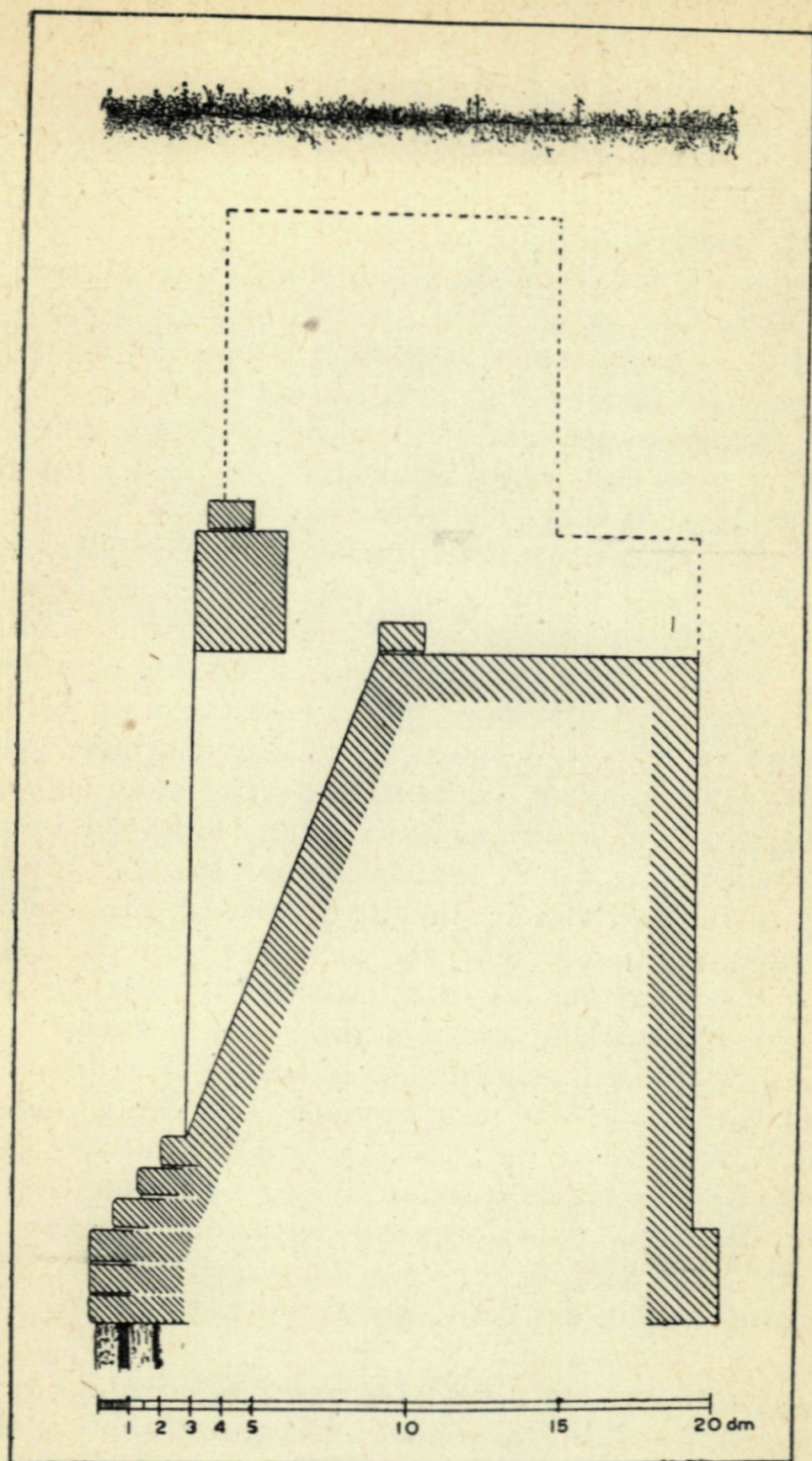
40. Doorsnede afvoerkoker.
